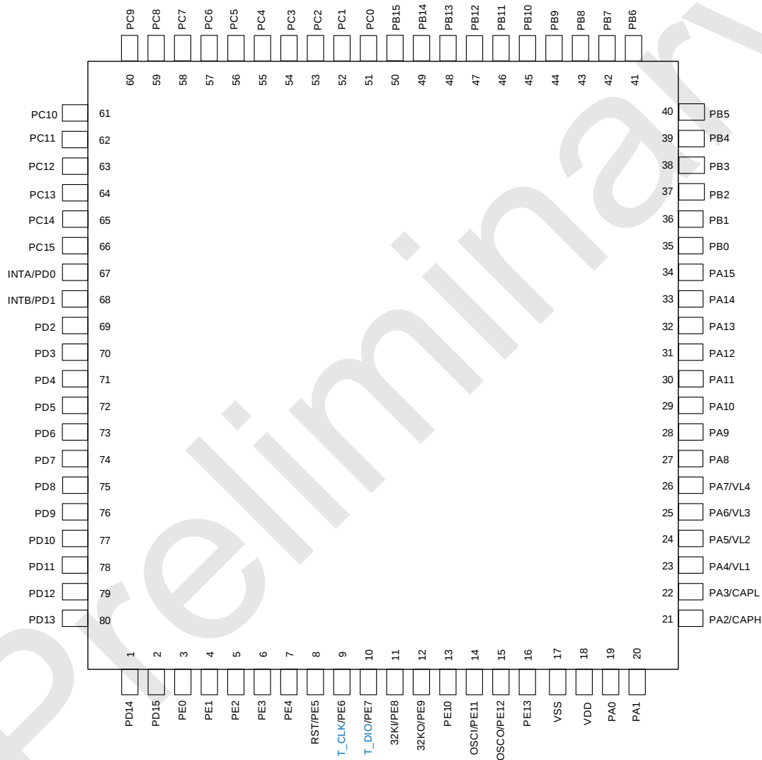
80PIN 管脚配置图 适用于 LQFP80
